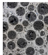
Konstruktions- leichtbeton (LC) mit einer dichten Matrixstruktur
