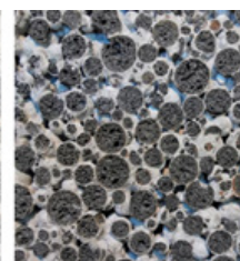
LAC mit offener Porenstruktur
